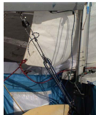
Figura 6 - ej. de sistema de trapa
