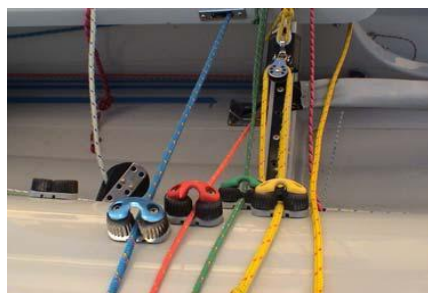
Figura 21 –trapa, cunningham de la mayor, carro del foque y carro de la mayor, colocados delante del caña
